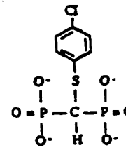
Tiludronate
